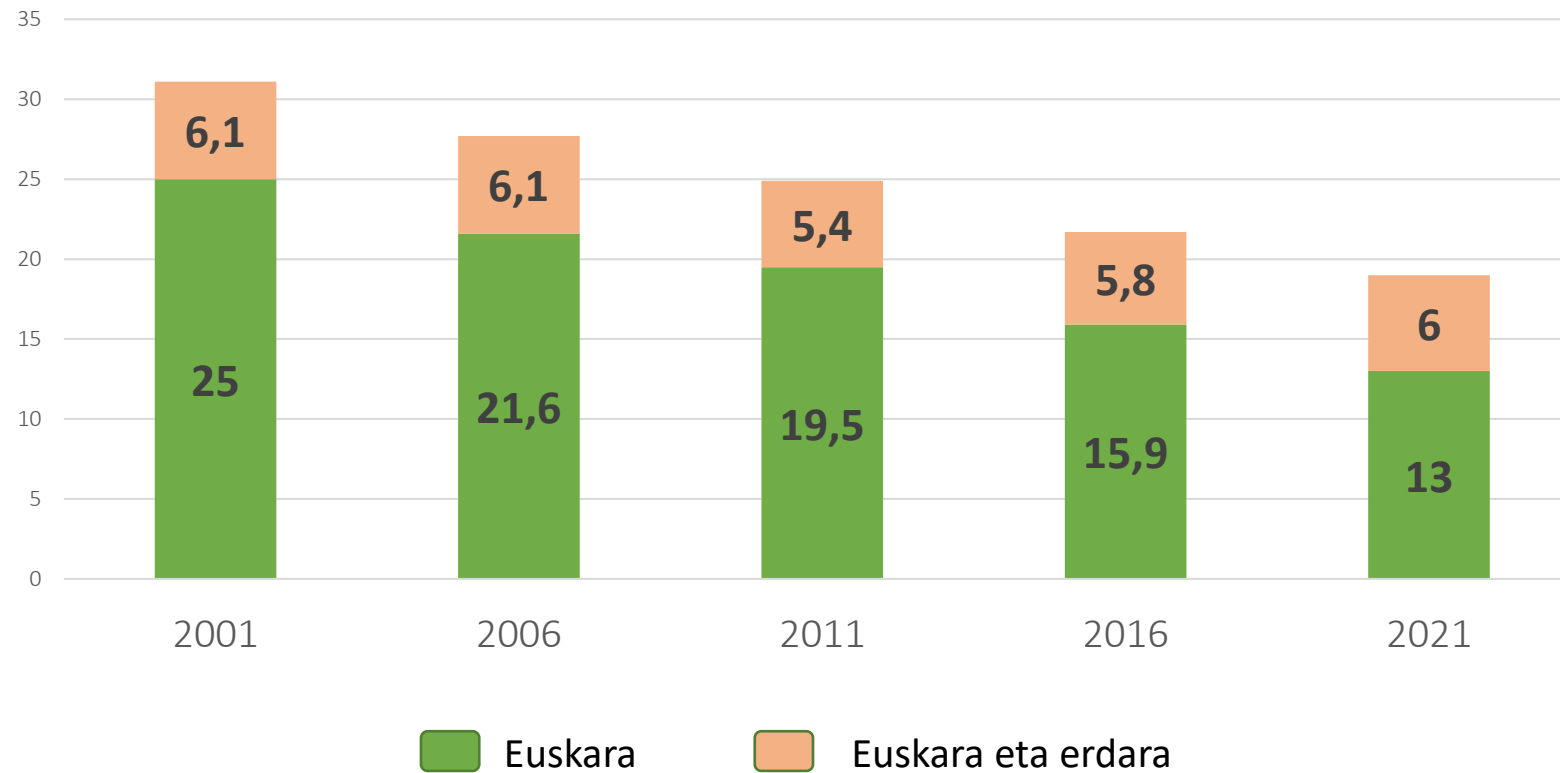
Lehen hizkuntzaren bilakaera (2001-2021). Iparraldea (%)
