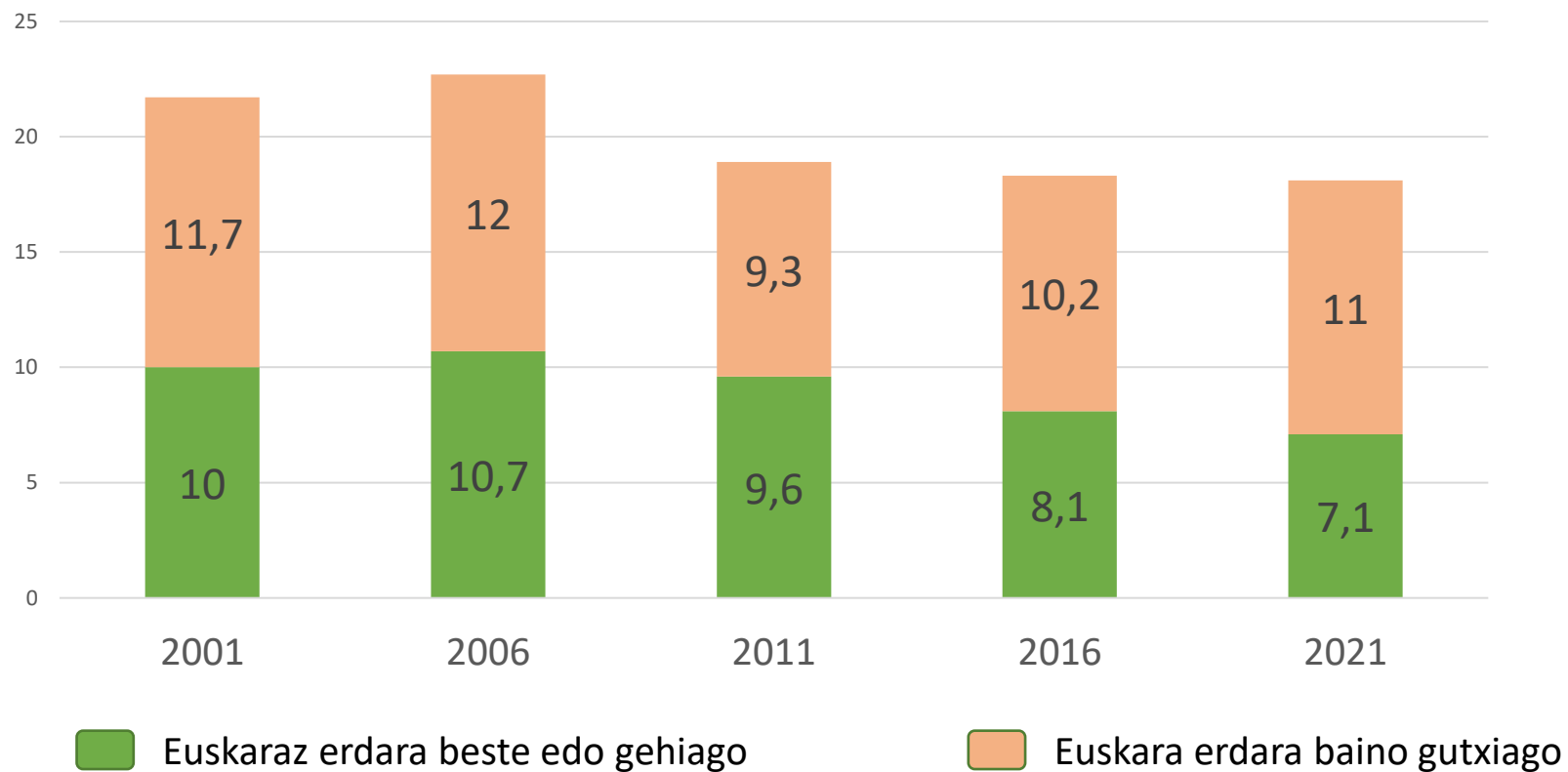
Euskararen erabileraren bilakaera, 2001-2021. Iparraldea (%)
