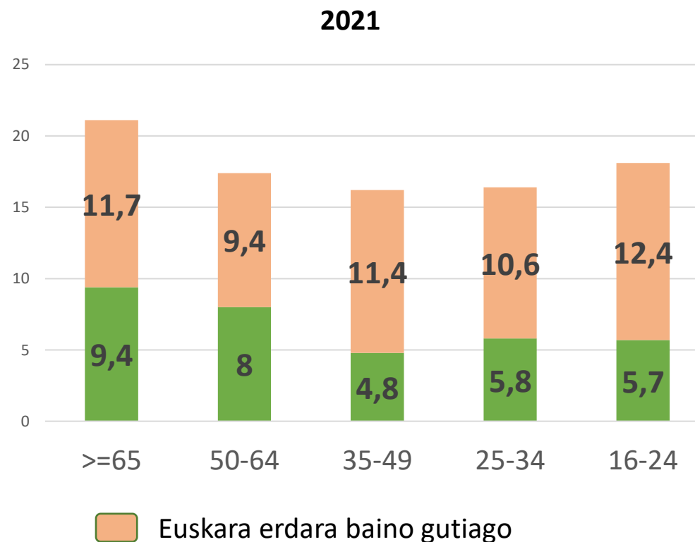
Euskararen erabileraren bilakaera adinaren arabera, 2011-2021. Iparraldea (%)
