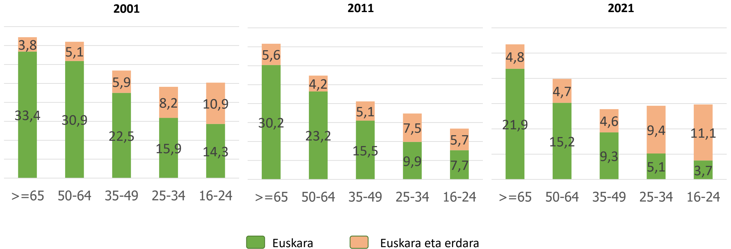
Lehen hizkuntza adinaren arabera, 2001 eta 2021. Iparraldea (%)
