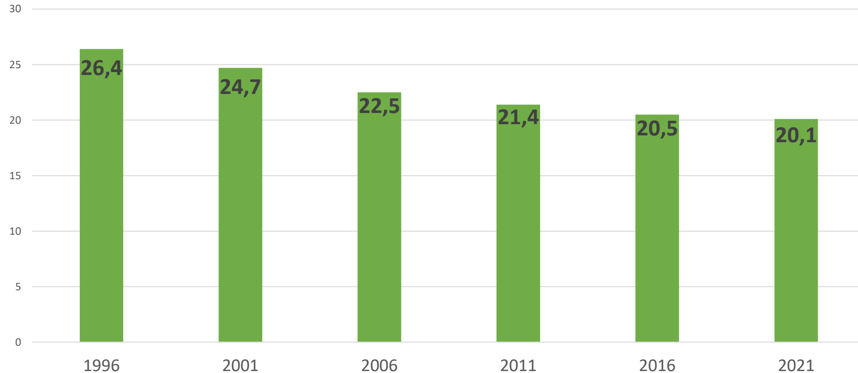
Euskaldunen proportzioaren bilakaera 1996tik 2021ra (%)
